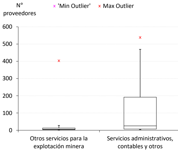
Fig. 14: Cantidad de proveedores de servicios externos varios OPEX
