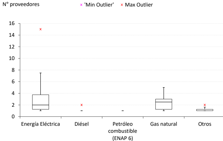
Fig. 5: Cantidad de proveedores de energía eléctrica y combustibles OPEX
