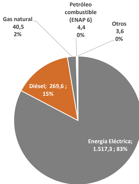
Fig. 4: Distribución gasto en energía eléctrica y combustibles OPEX (MMUS$; %)
