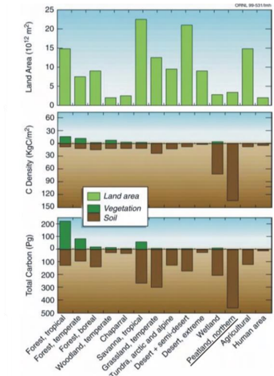
Figura 2-4. Área, densidad de carbono y carbono total en suelo y vegetación para los principales biomas terrestres.
