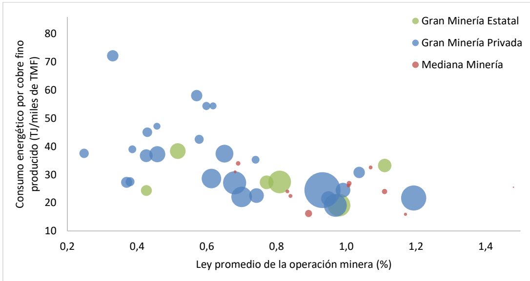
Figura 12 Consumo energético por cobre fino producido versus ley promedio del mineral por operación minera, 2019
