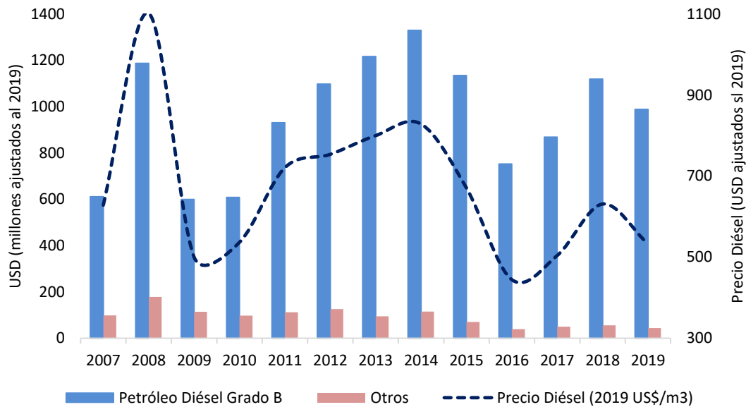
Figura 25 Gasto agregado en combustibles de la minería del cobre, 2007-2019
