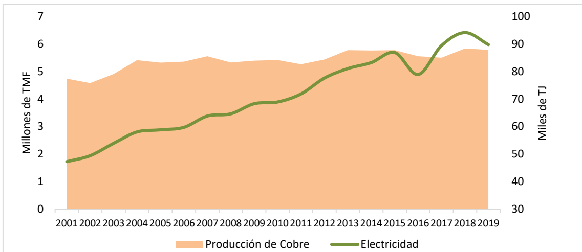
Figura 18 Consumo de energía eléctrica en la minería del cobre, 2001-2019
