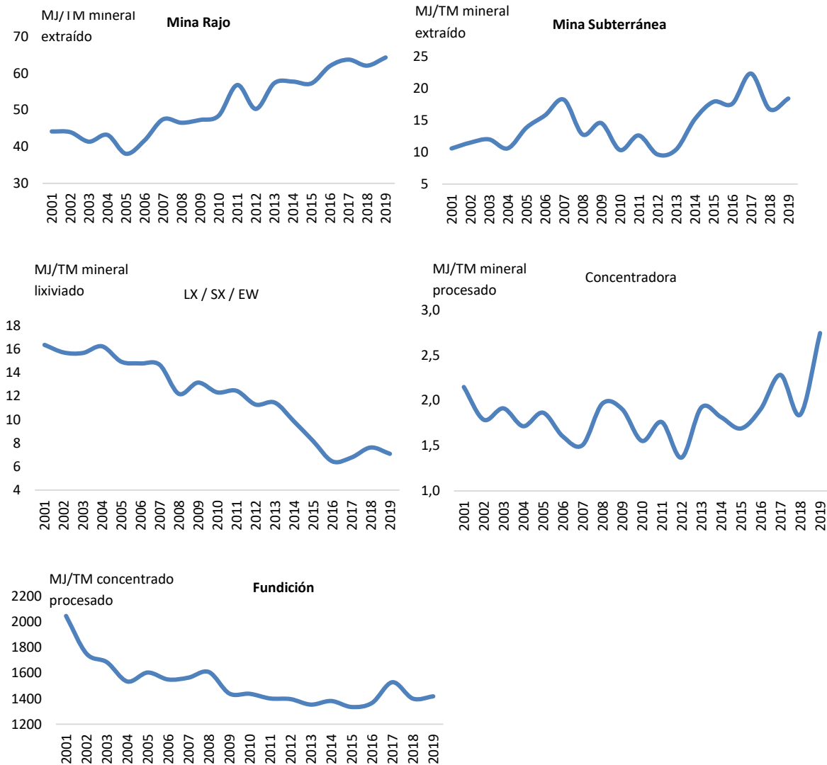
Figura 17 Consumos unitarios de combustibles por tonelada de material procesado, 2001-2019
