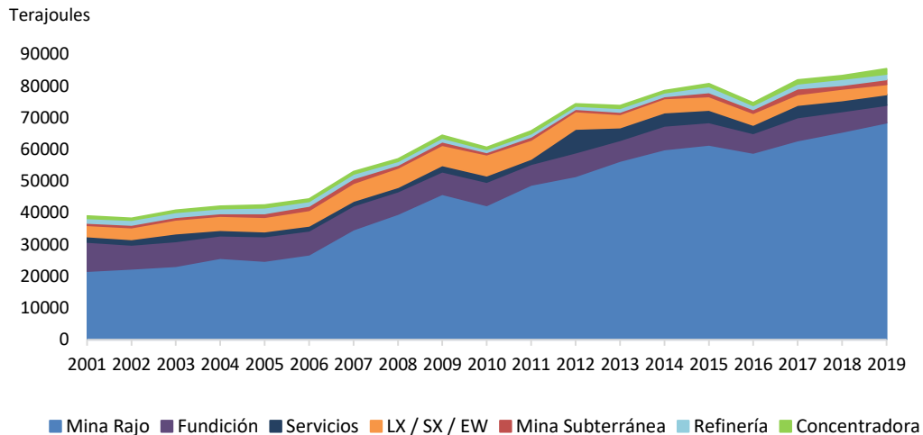
Figura 15 Evolución en el consumo de combustibles por proceso, 2001 – 2019
