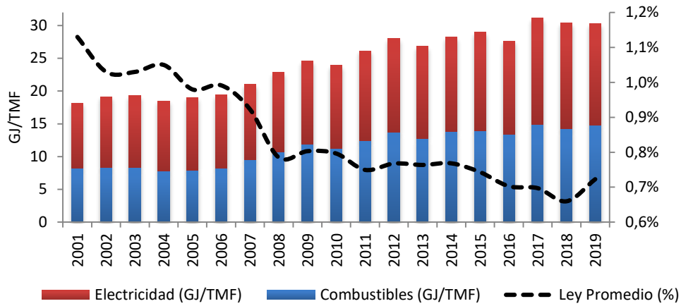
Figura 11 Evolución del consumo unitario de energía y leyes a nivel nacional, 2001-2019
