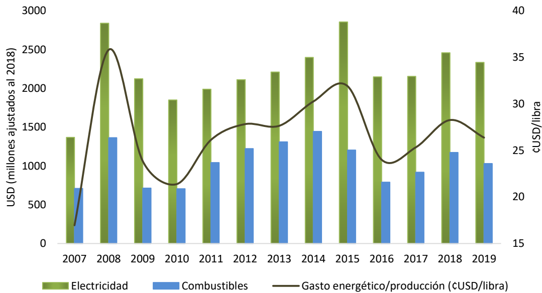
Figura 26 Gasto energético agregado de la minería del cobre, 2007-2019
