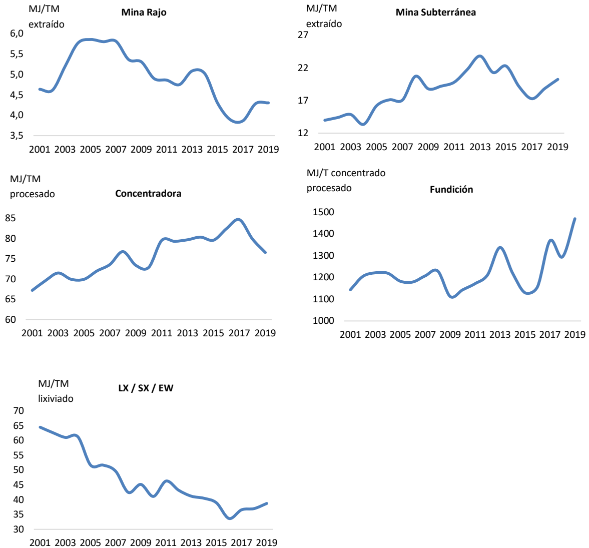
Figura 23 Consumo unitario de electricidad por tonelada de mineral extraído/procesado (MJ/TM), 2001-2019
