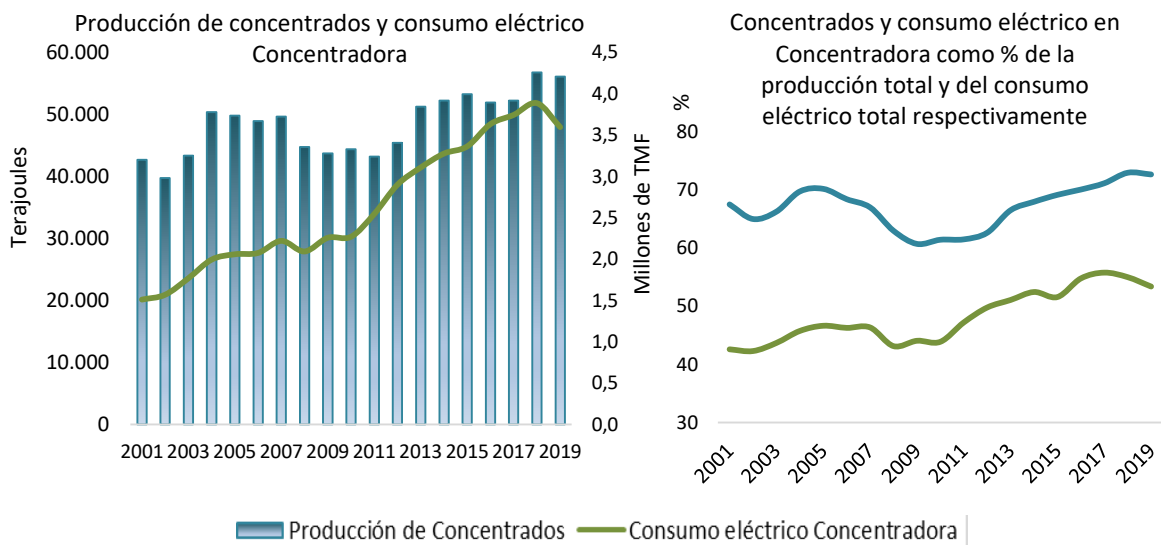
Figura 20 Producción de concentrados y consumo eléctrico en Concentradora en la minería del cobre, 2001 - 2019
