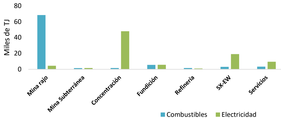
Figura 6 Consumo de electricidad y combustibles por procesos en la minería del cobre, 2019
