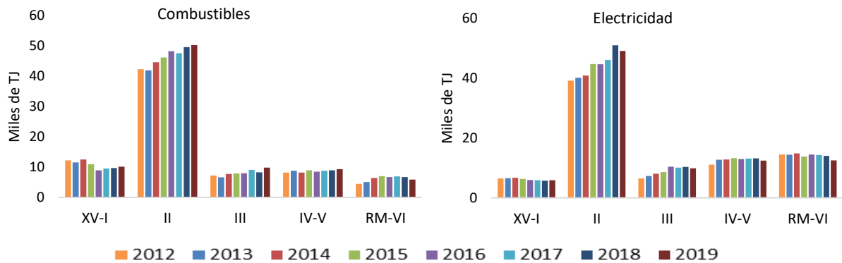
Figura 9 Consumo de energía en la minería del cobre por región, 2012-2019
