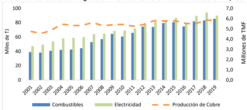
Figura 3 Consumos Totales de Energía de la Minería del Cobre vs Producción de Cobre Fino, 2001-2019
