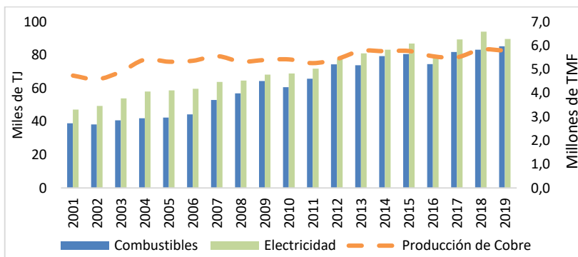
Consumo energético y producción cuprífera, 2001-2019
