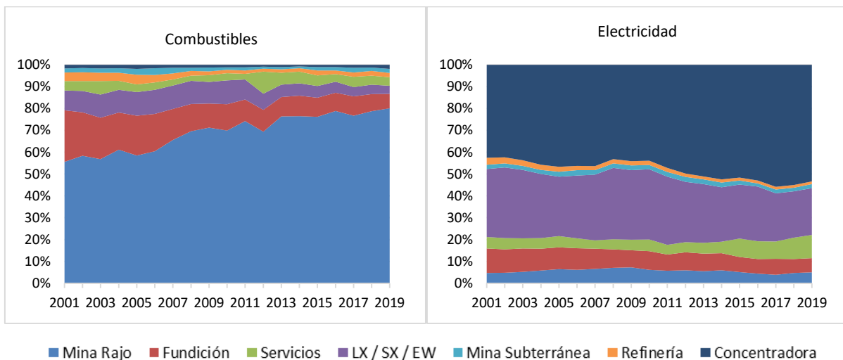
Figura 7 Evolución en la participación (%) por proceso en el consumo de combustibles y electricidad, 2001-2019
