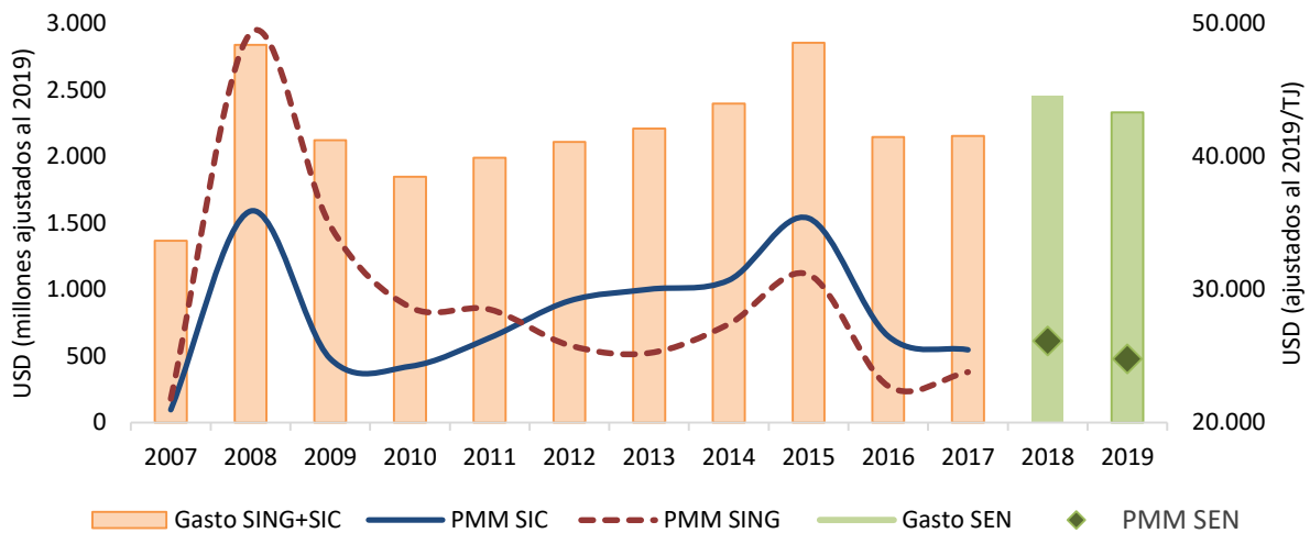
Figura 24 Gasto agregado en electricidad de la minería del cobre, 2007-2019
