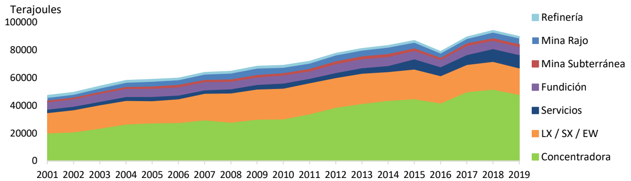
Figura 19 Evolución en el consumo de electricidad por proceso, 2001 - 2019
