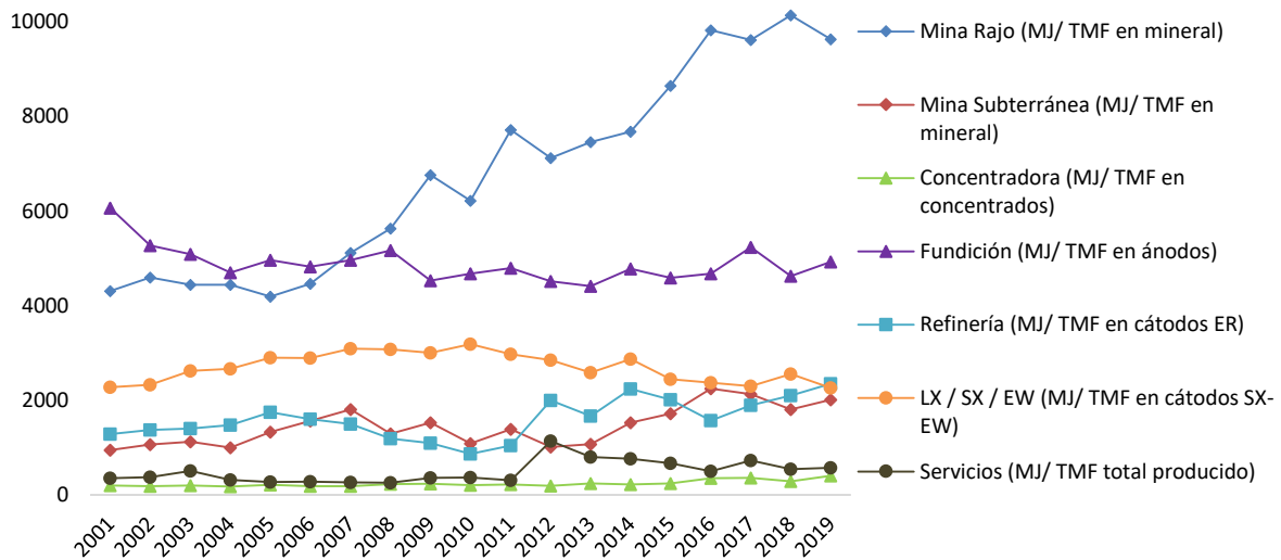
Figura 16 Consumos unitarios de combustibles por tonelada de cobre fino contenido (MJ/TMF). 2001-2019
