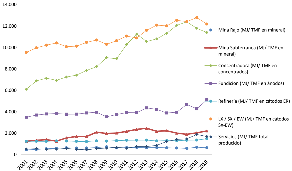
Figura 22 Consumo unitario de electricidad por tonelada de cobre fino contenido (MJ/TMF), 2001-2019
